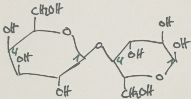
Lactose
