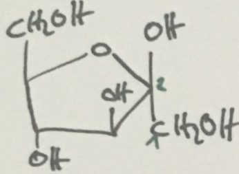
D-Fructose
