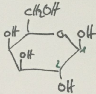
D-Galactose
