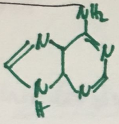
Adenin
