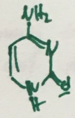
Cytosin
