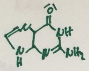
Guanin
